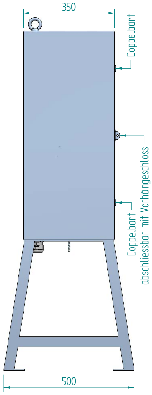
Schema Art.Nr. 231124
